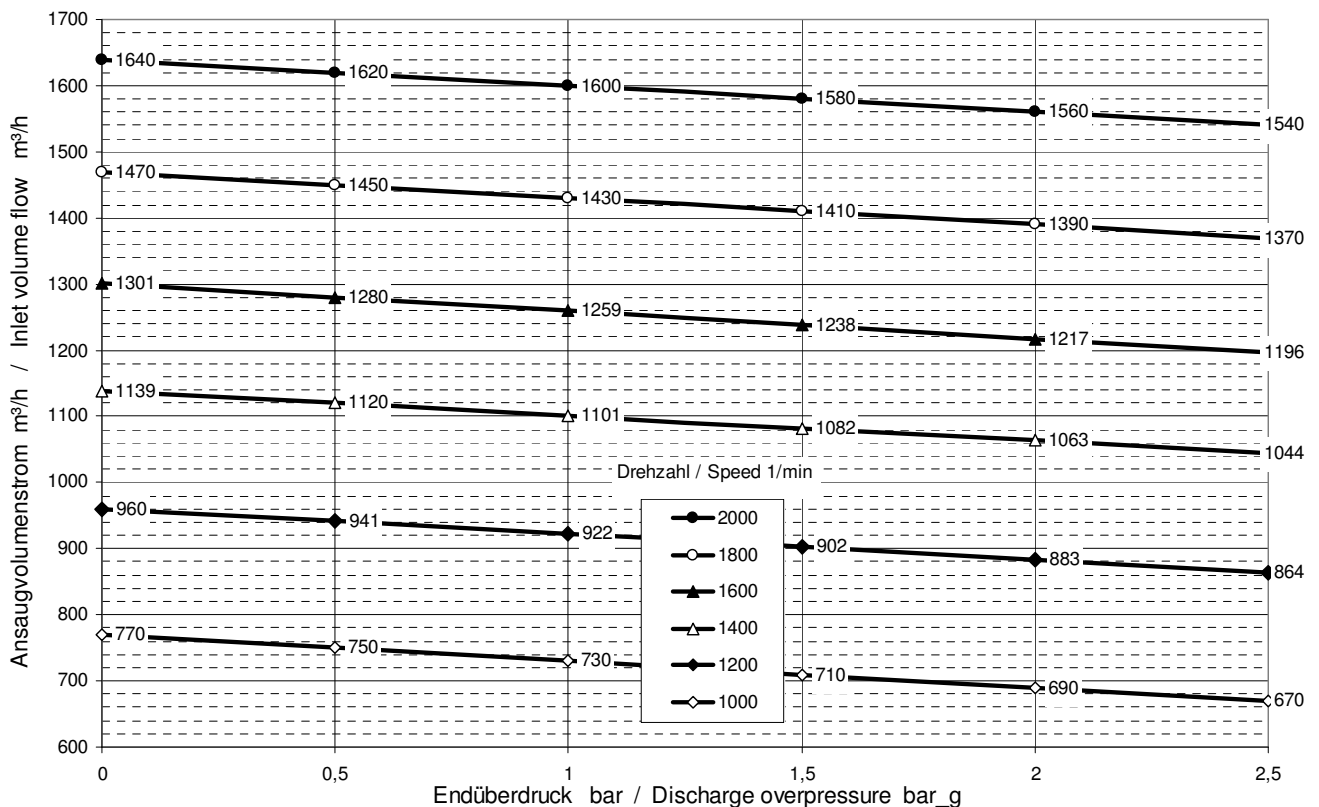
Ansaugvolumenstrom / Inlet volume flow
