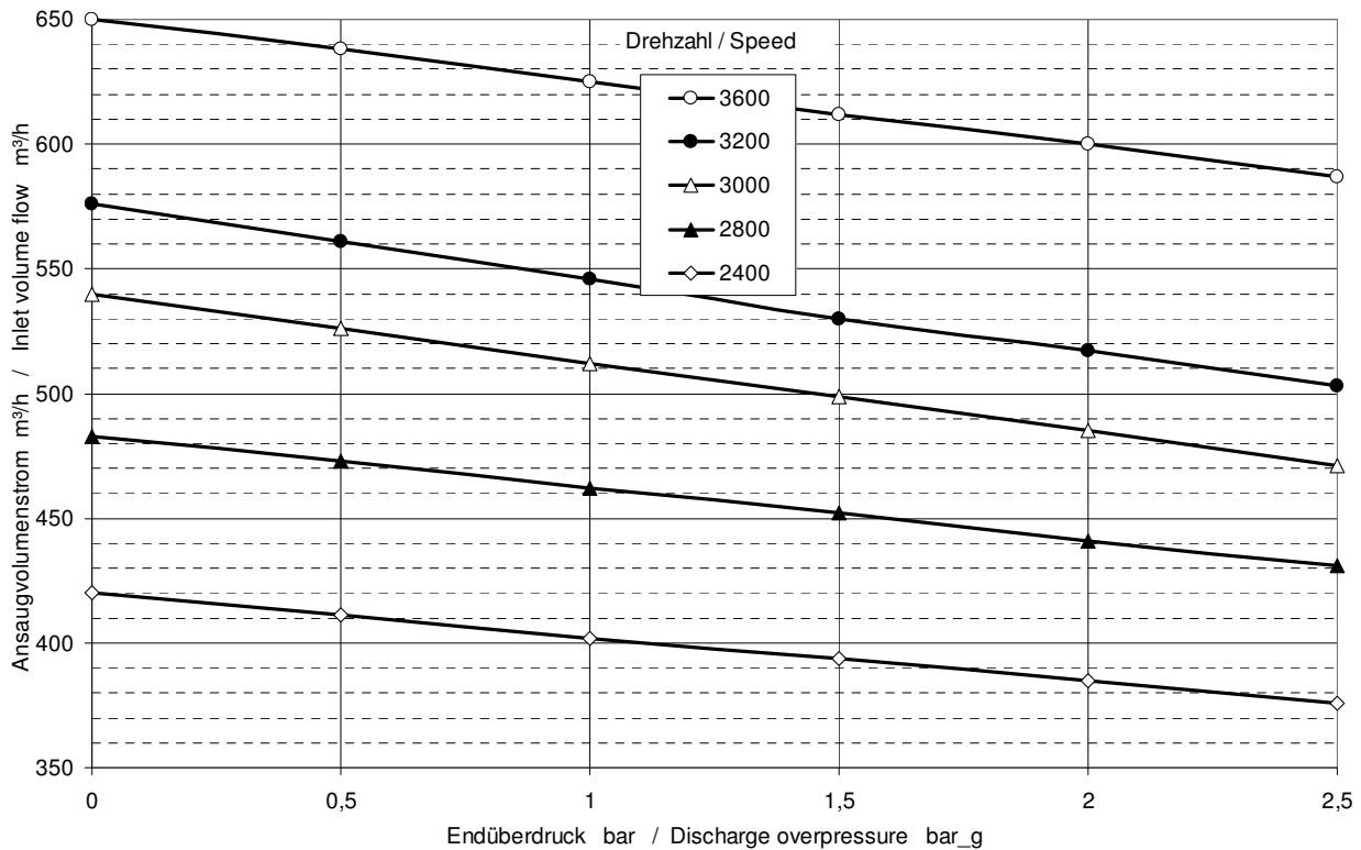
Ansaugvolumenstrom / Inlet volume flow
